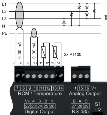
Anschlussbeispiel Multifunktionskanäle für die Differenzstrom- und Temperaturmessung
